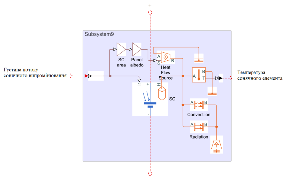
Рис. 3. Блок Solar Cell з удосконаленою тепловою схемою
