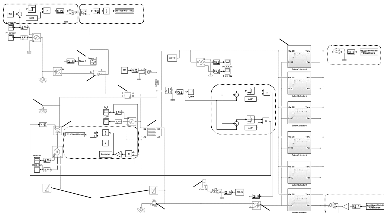
Рисунок 1. Імітаційна модель системи сонячного гарячого водопостачання
