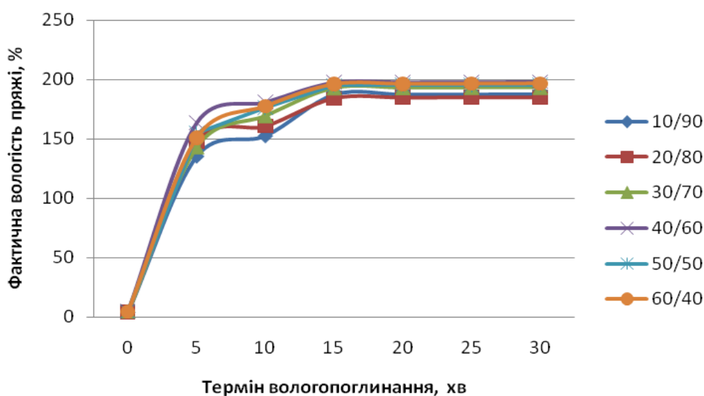
Рис. 4.11. Залежність фактичної вологості змішаної пряжі з волокон льону олійного та лавсану від терміну вологопоглинання
