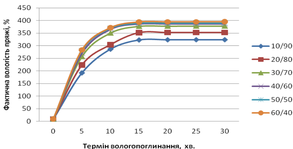
Рис. 4.9. Залежність фактичної вологості змішаної пряжі з волокон льону олійного та бавовни від терміну вологопоглинання
