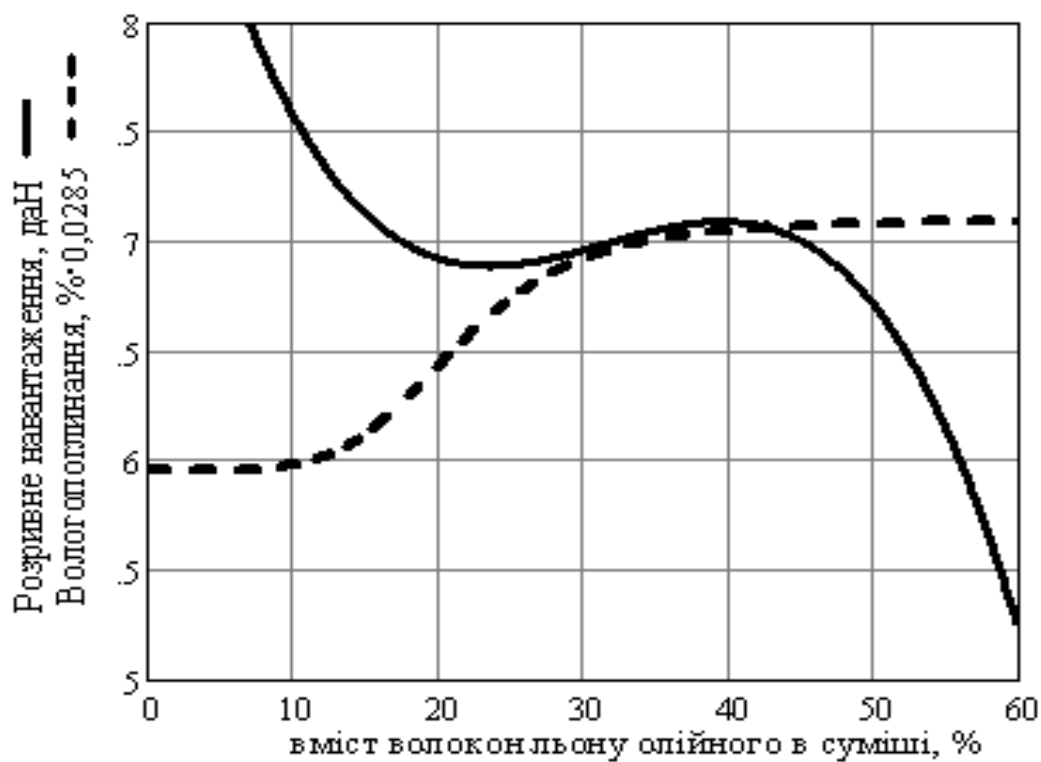
Рис. 4.18. Залежність вологопоглинання та розривного навантаження від вмісту волокон льону олійного в льоно-нітроновій пряжі
